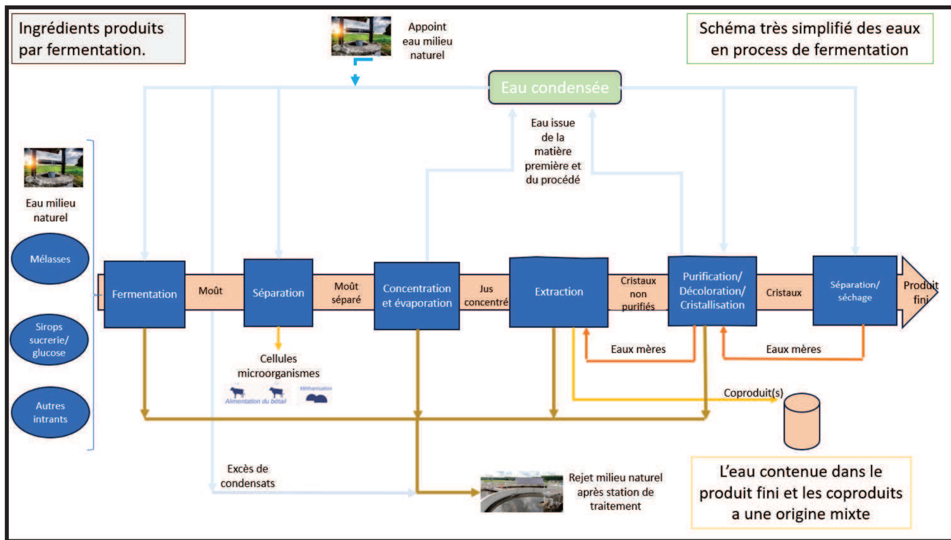
Process n°6 : Production d'ingrédients par fermentation
